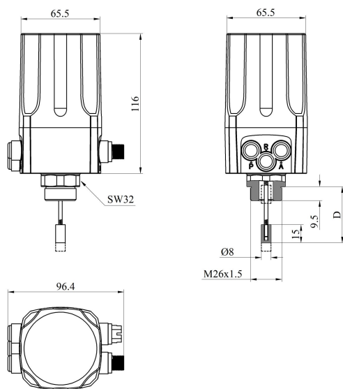
分体式传感器尺寸
