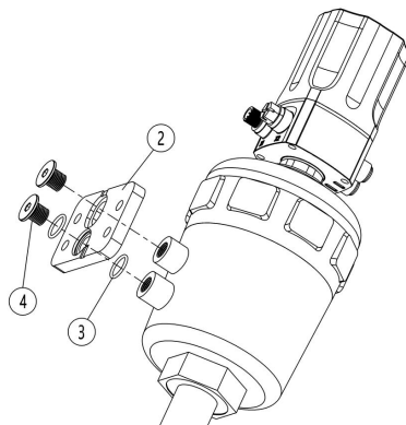
固定安装板
