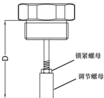
调节D值
